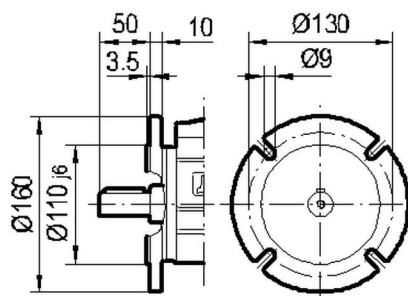
II Ø160
