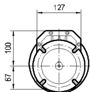
III Ø200
