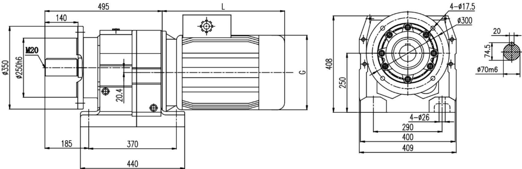
С Выходным фланцем Ø350
