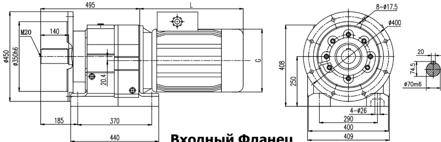
С Выходным фланцем Ø450
