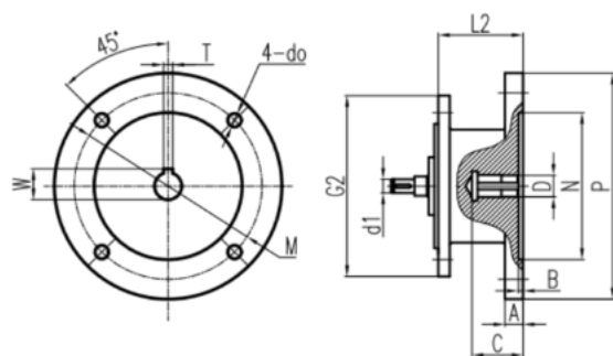
63B5~200B5
