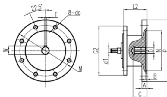
225B5~315B5
