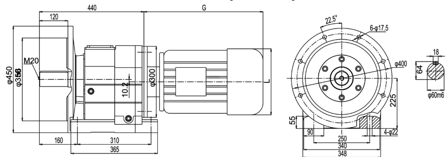
С выходным фланем ф450
