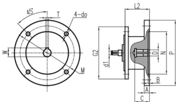
63B5~200B5
