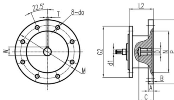
225B5~315B5
