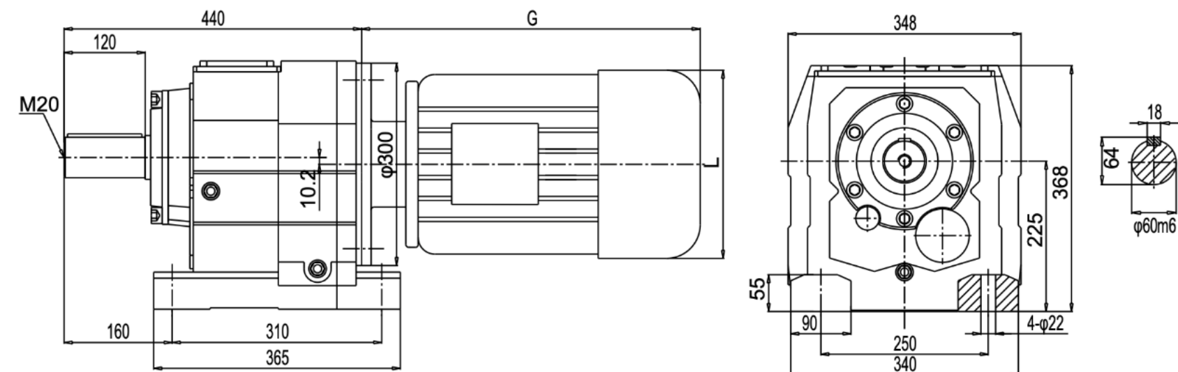
С выходным фланем ф350
